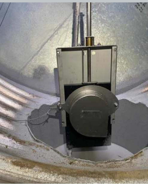
Vanne de confinement avec vortex
